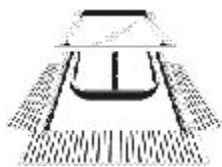
Universaldachfenster verzinkt, 45 x 55 cm inkl. Glas (ESG) (Schornsteinfeger-Ausstieg nach DIN 18160)
